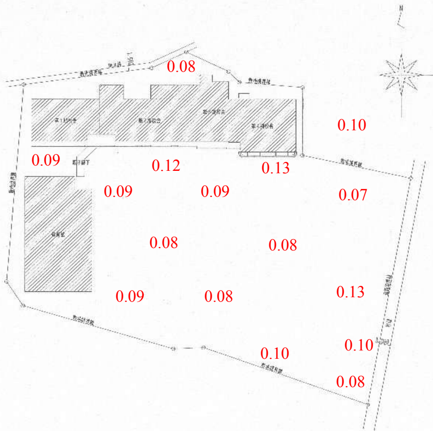
配置図 S=1/600
