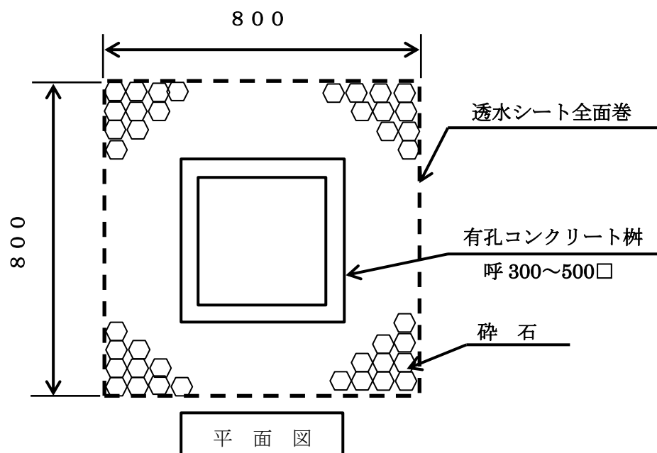
標準浸透枘構造図 (図1)
