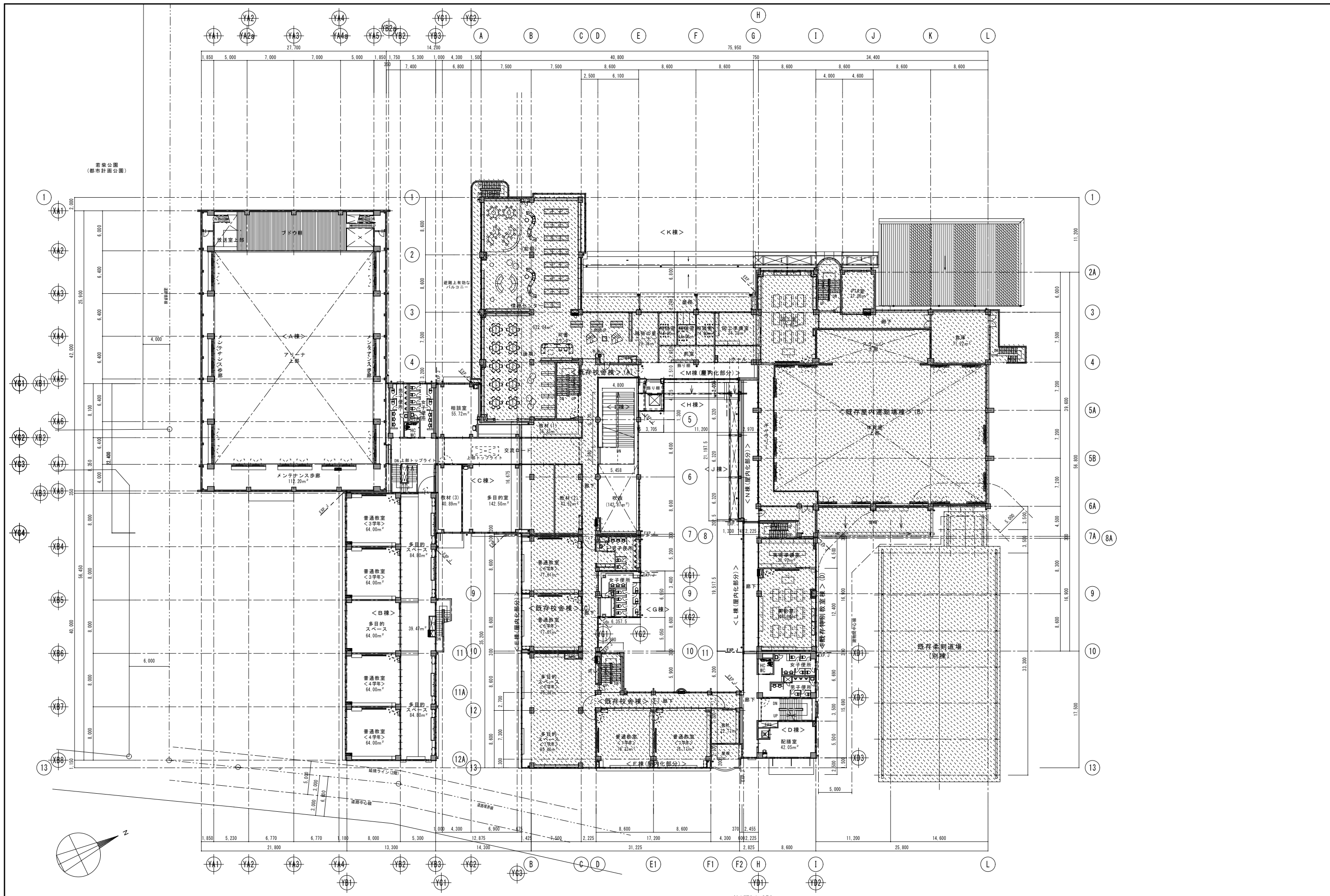
2階計画平面図 (A1版) 1:250 (A3版) 1:500
