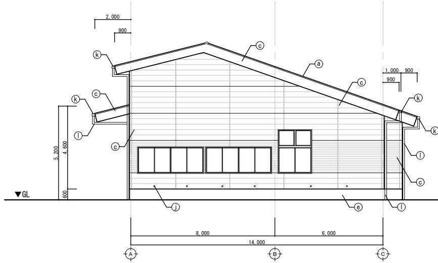
東立面図 S=1/75
