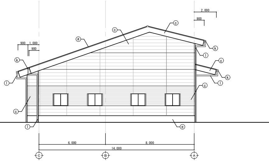
西立面図 S=1/75
