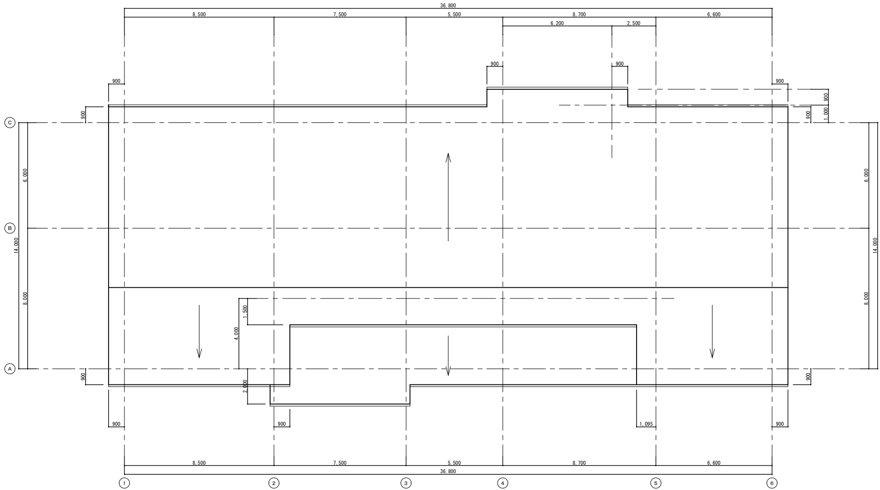
屋根伏図 S=1/75
