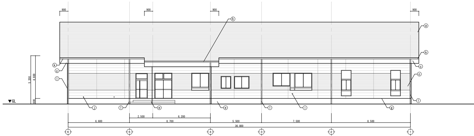
北立面図 S=1/75
